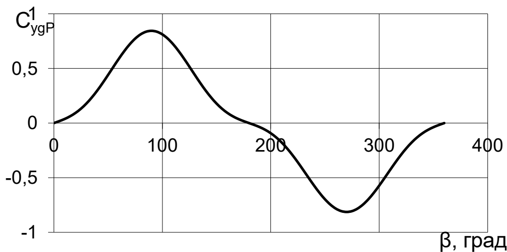
Рис. 2. Зависимость позиционного поперечного коэффициента гидродинамической силы в функции от угла дрейфа
