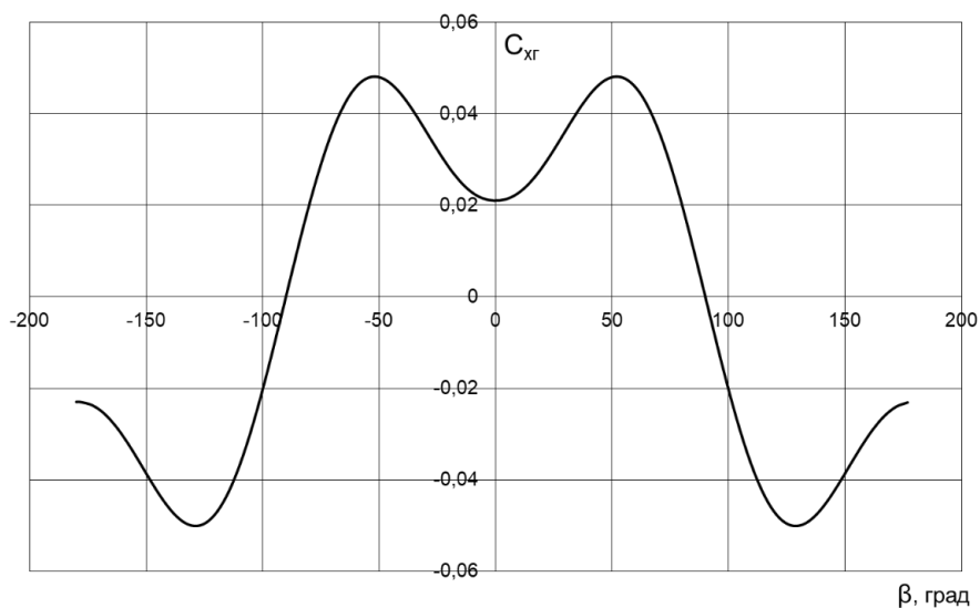
Рис. 1. Зависимость продольного гидродинамического коэффициента в функции от угла дрейфа
