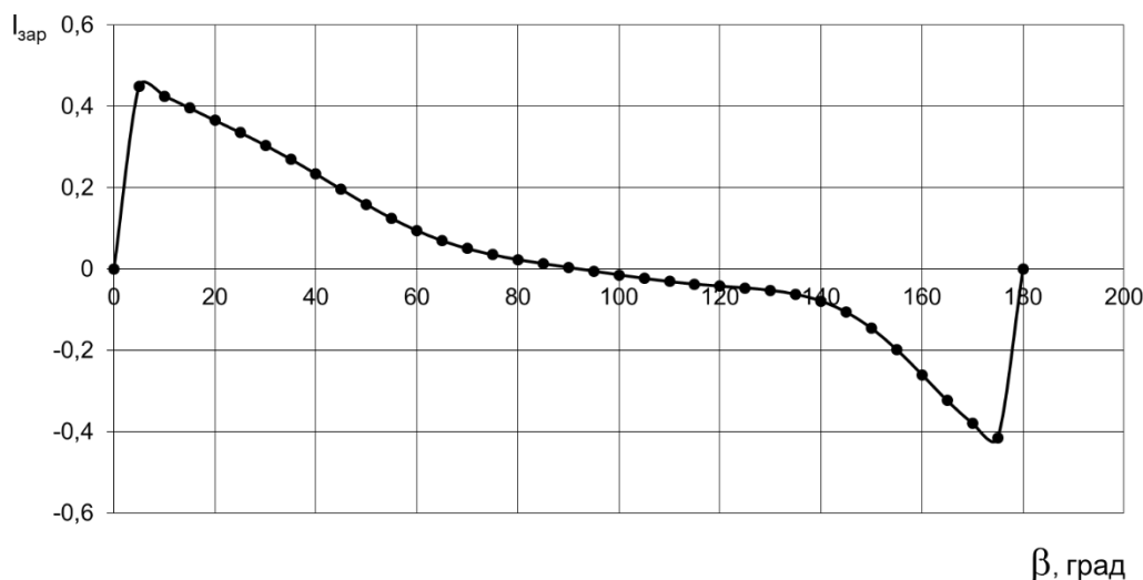
Рис. 4. Зависимость плеча позиционного момента в функции от угла дрейфа
