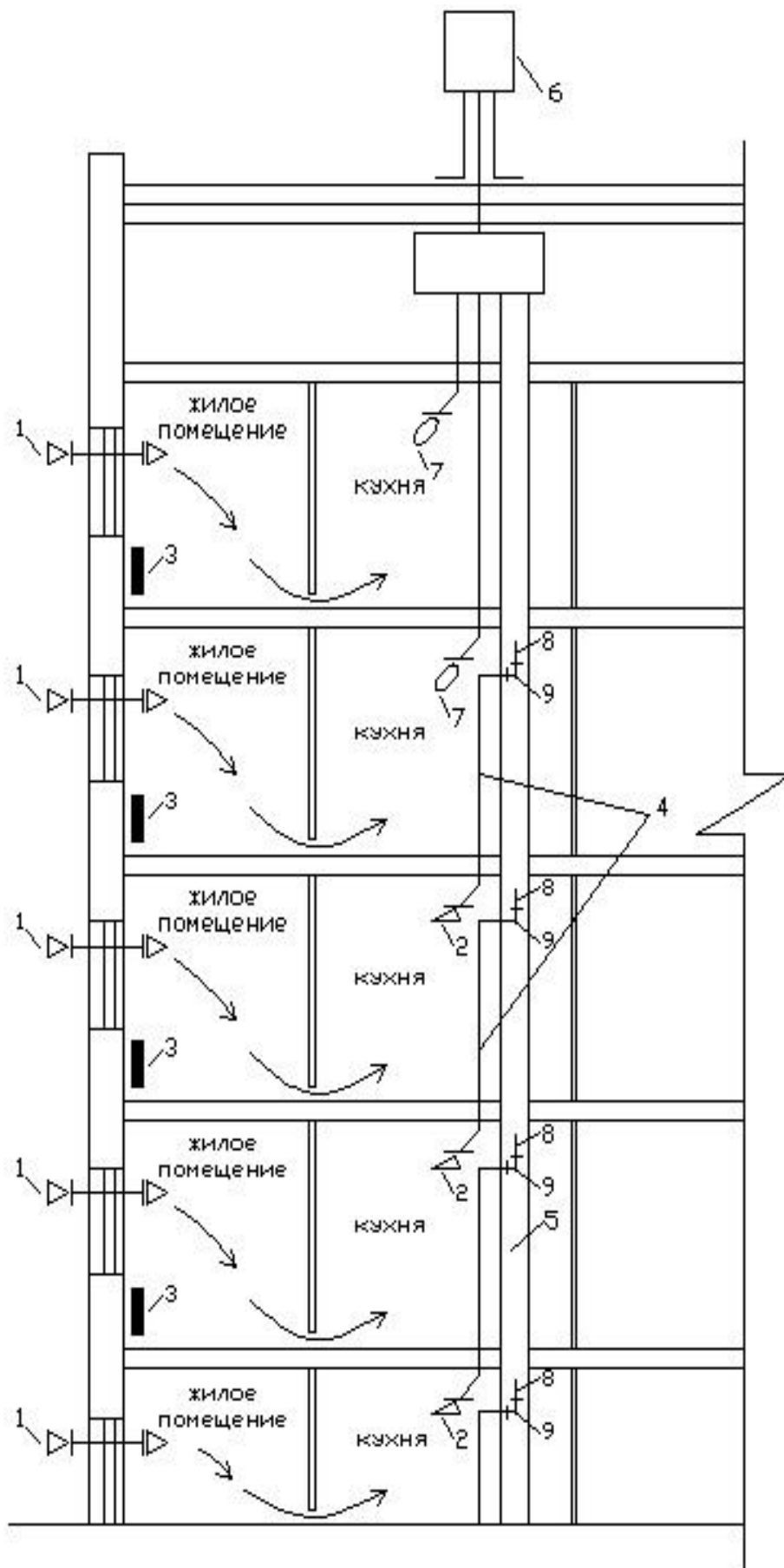
Рис. 1. Схема вентиляции жилого здания
