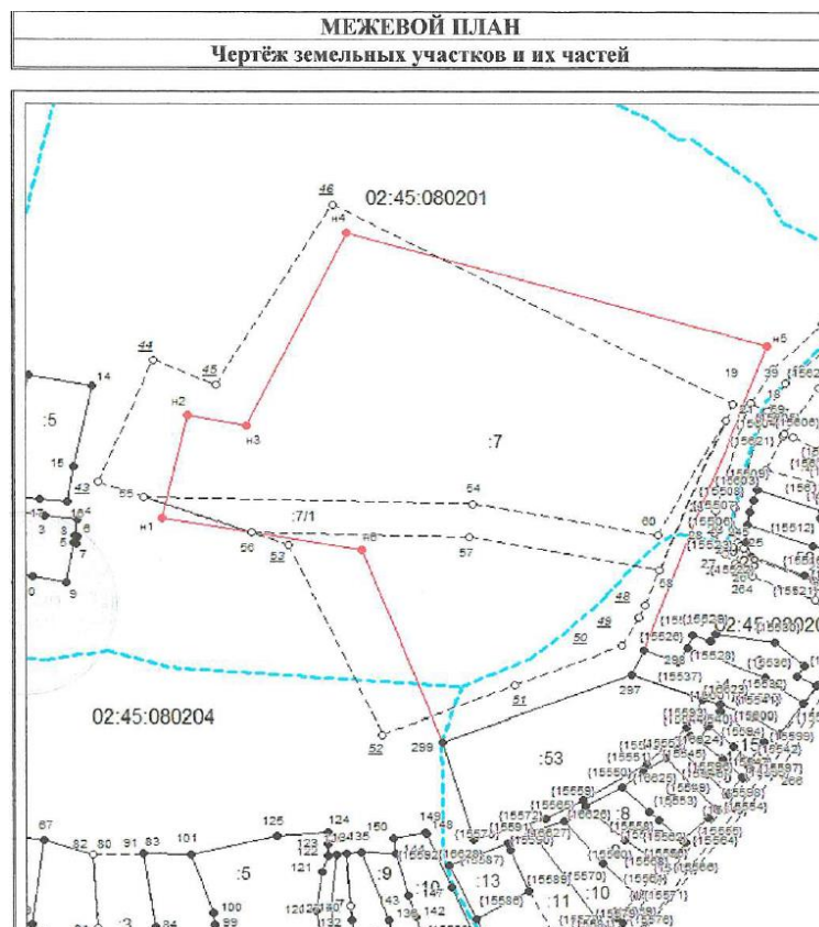
Рис. 2. Чертеж земельных участков и их частей
