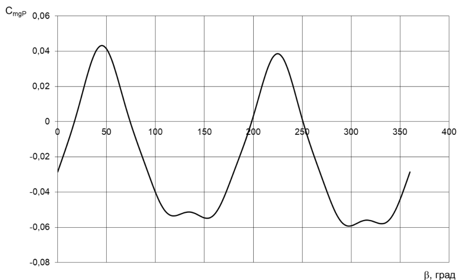
Рис. 3. Зависимость позиционного коэффициента момента в функции от угла дрейфа
