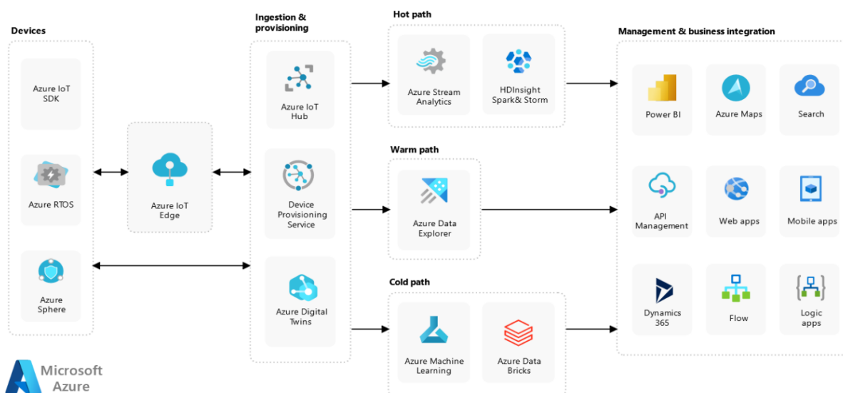
Рис.1.Архитектура Azure Digital Twins. [3]
