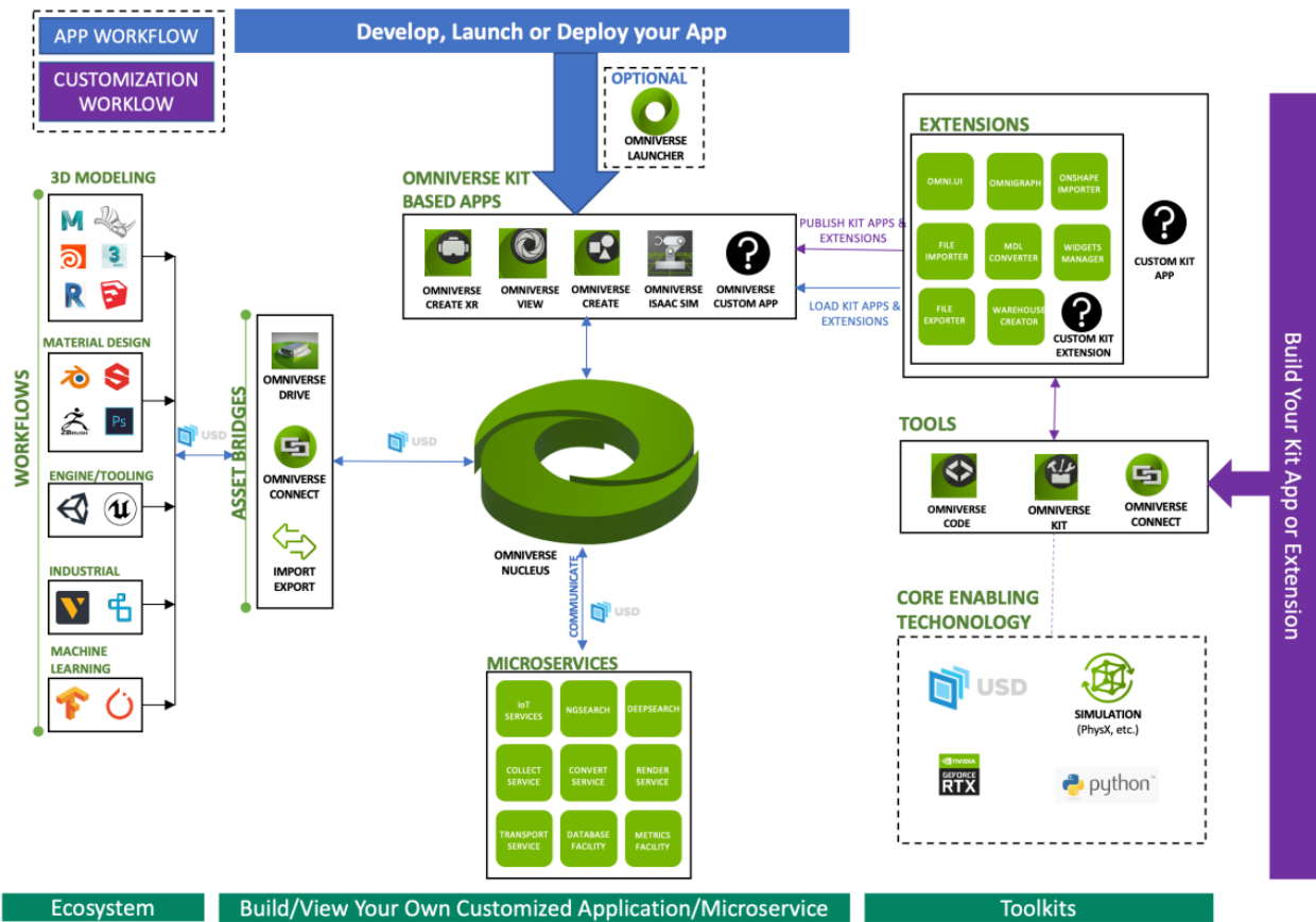
Рис. 2. Взаимодействие компонентов в NVIDIA Omniverse. [5]
