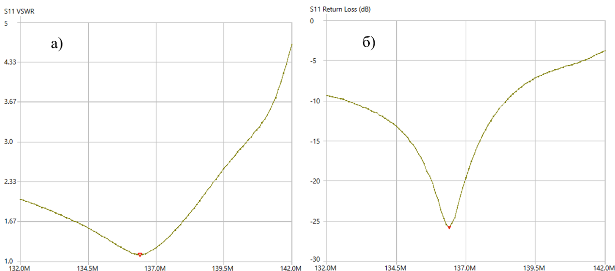
Рис. 2. Характеристики антенны а) КСВ б) возвратные потери
