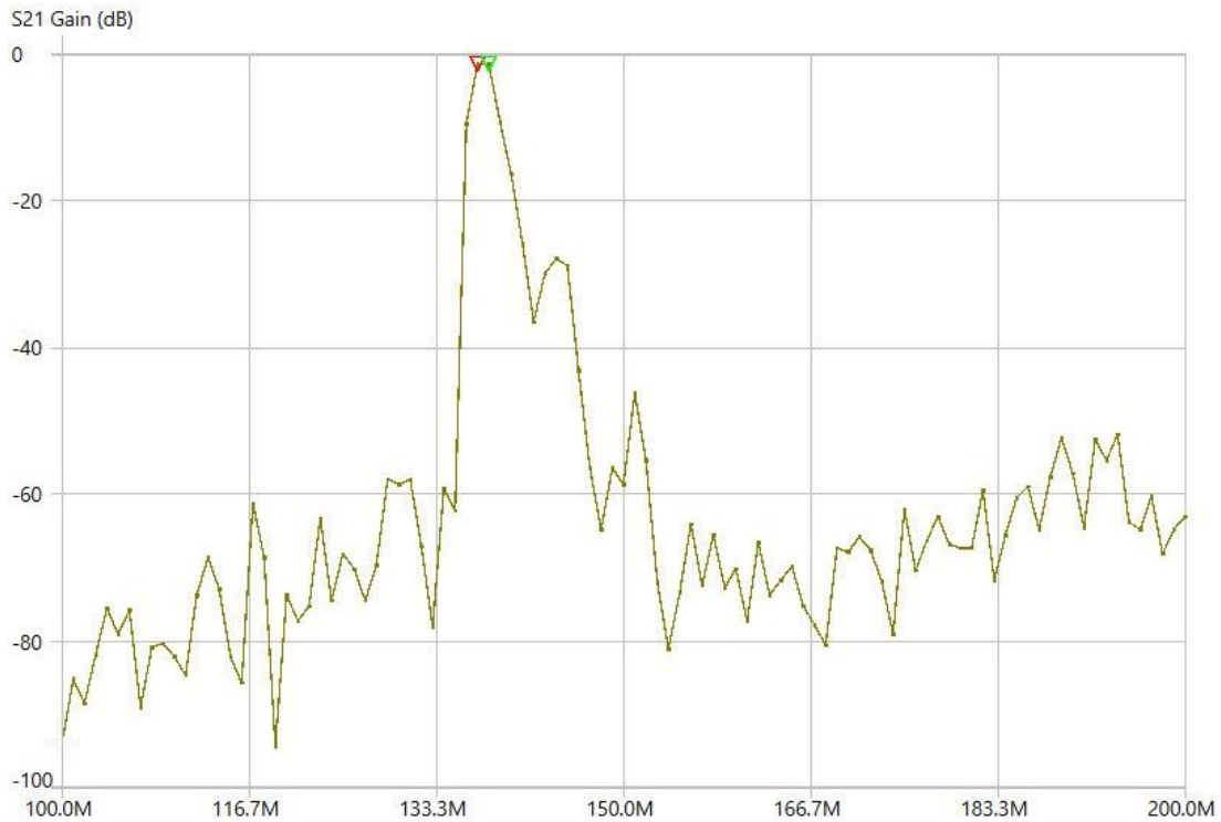
Рис. 3. Характеристика band pass фильтра
