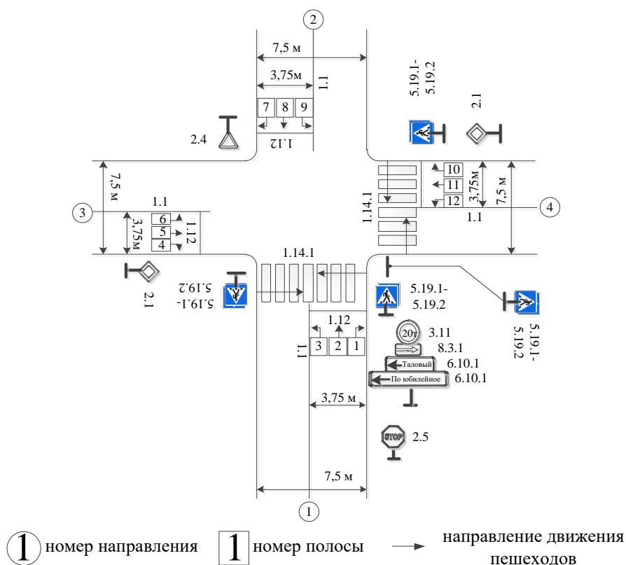
Рис. 3. Геометрические параметры пересечения ул. Суворовская – ул. Победная
