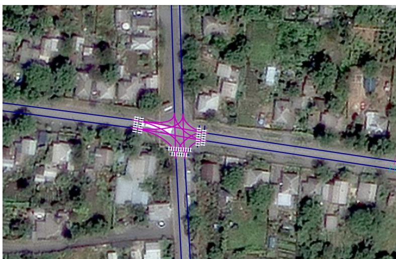
Рис. 4. Схема соединительных отрезков на пересечении ул. Суворовская – ул. Победная
