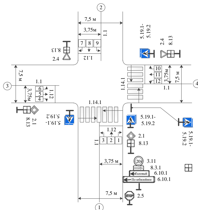
Рис. 10. Предлагаемая схема организации дорожного движения
