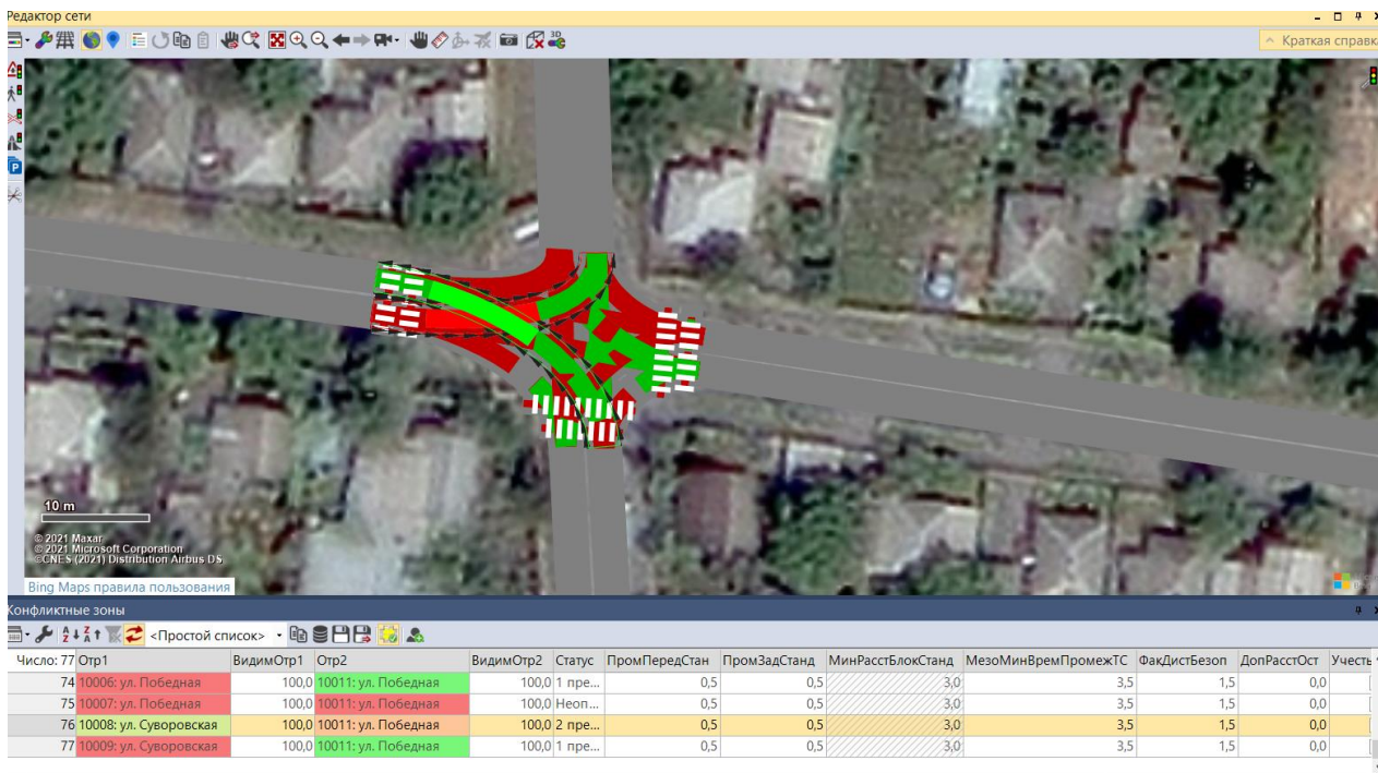
Рис. 7. Схема конфликтных зон на пересечении
