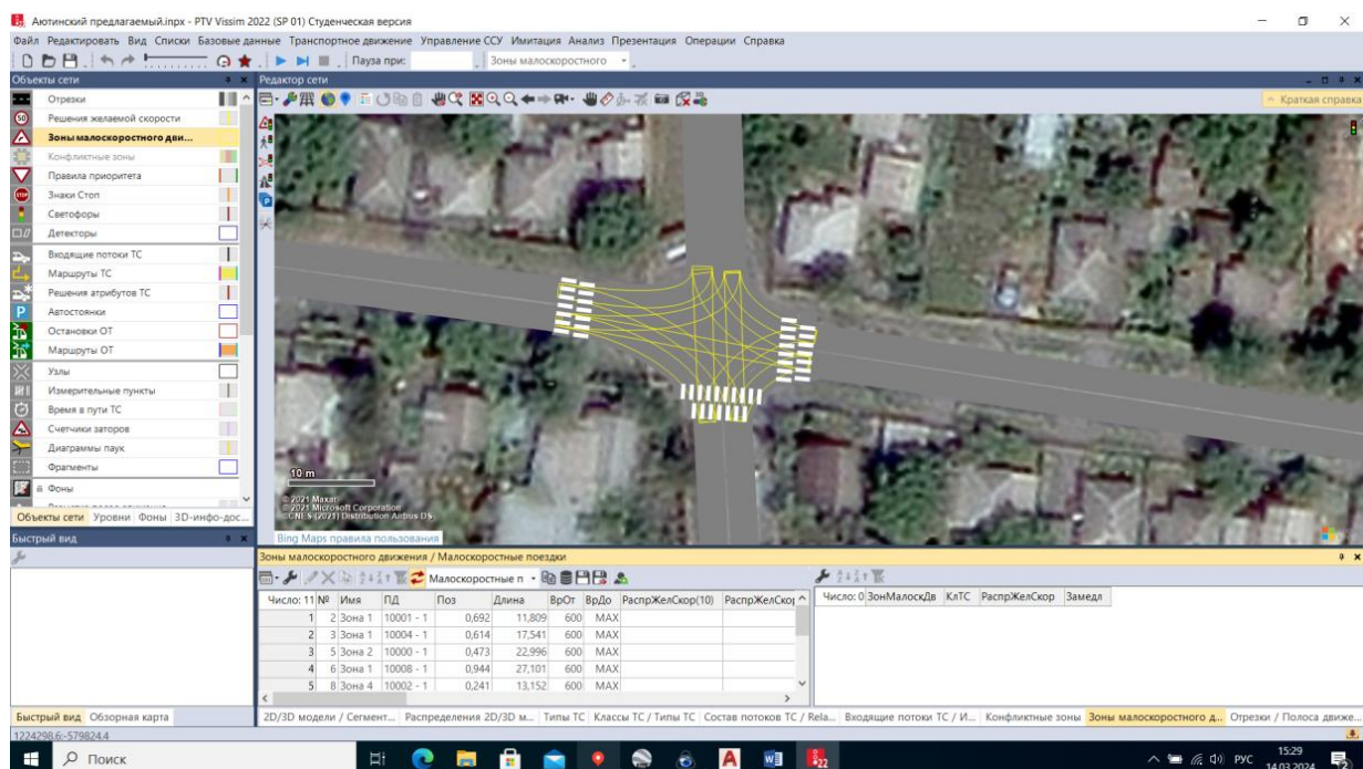
Рис. 8. Схема зон малоскоростного режима на пересечении ул. Суворовская – ул. Победная
