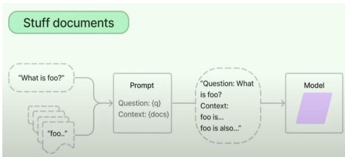
Рис. 2. Схема формирования ответа типа Stuff
