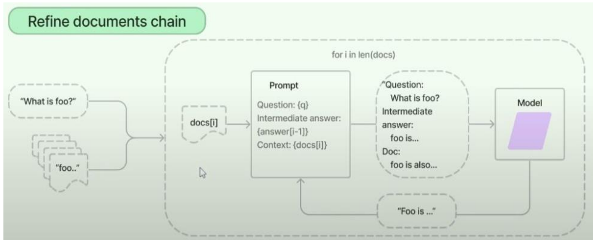
Рис. 3. Схема формирования ответа типа Refine
