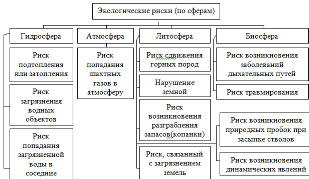
Рис. 1. Экологический риски
