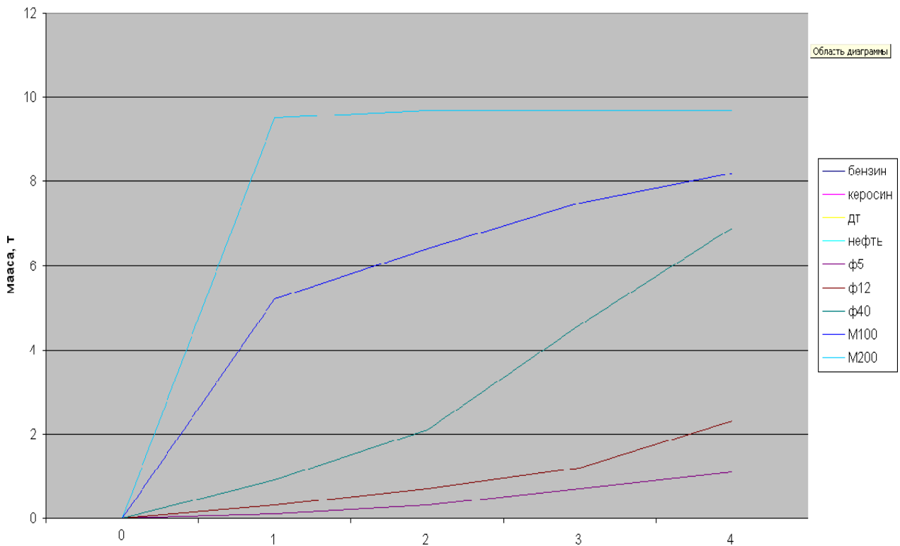
Рис. 3. Количество утонувшего нефтепродукта
