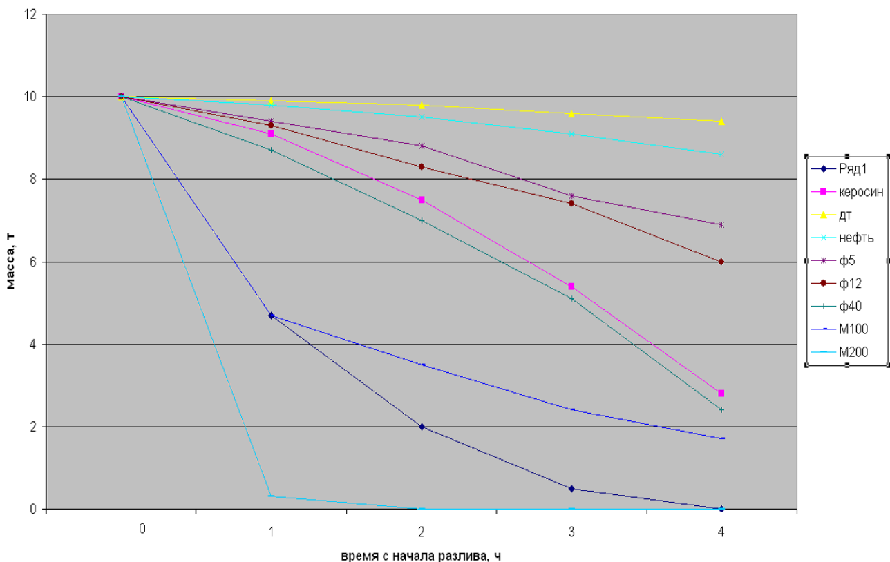
Рис. 1. Количество нефти на плаву
