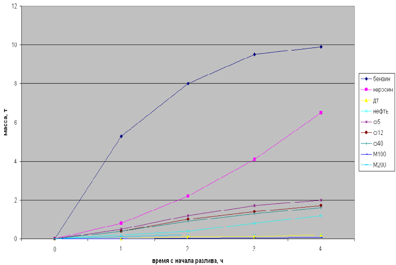
Рис. 2. Количество испарившейся нефти
