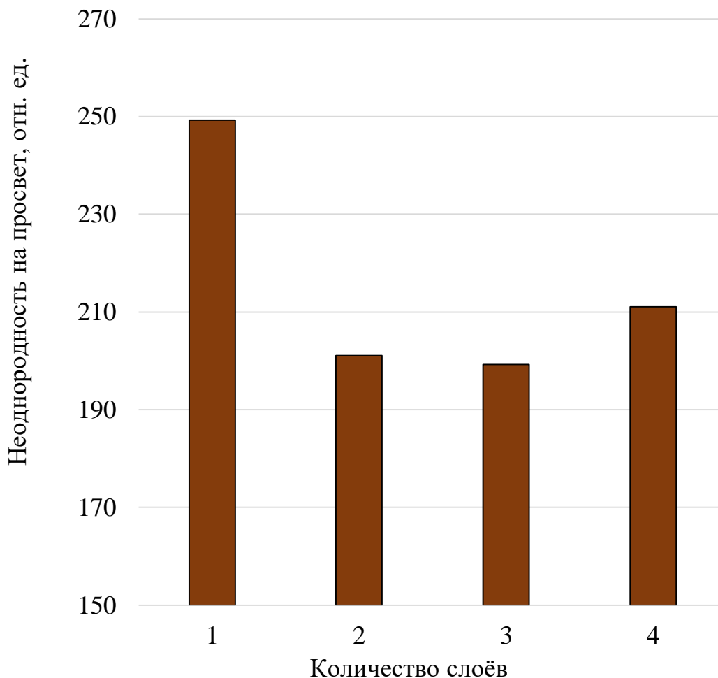
Рис. 2. Неоднородность на просвет образцов, изготовленных из вторичных волокон, содержащихся в гофрокартоне
