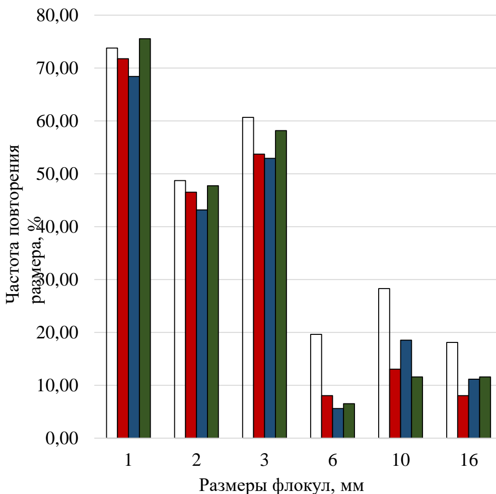
Рис.3. Размеры флоккул образцов, произведённых из вторичных волокон, содержащихся в гофрокартоне с различным количеством слоёв: □ – один слой; ■ – два слоя; ■ – три слоя; ■ – четыре слоя
