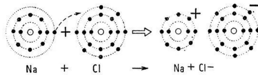
Рис. 1. Разложение на ионы NaCl
