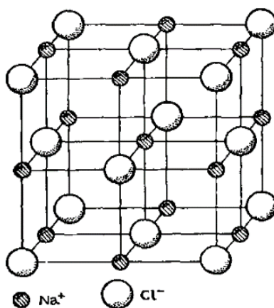
Рис. 2. Ионно-кристаллическая решетка NaCl
