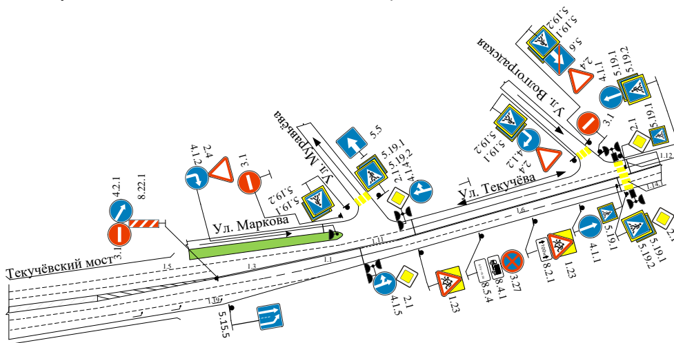
Рис. 6 – Предлагаемая схема ОДД на перегоне по ул. Текучёва от Текучёвского моста до пересечения с ул. Волгоградской
