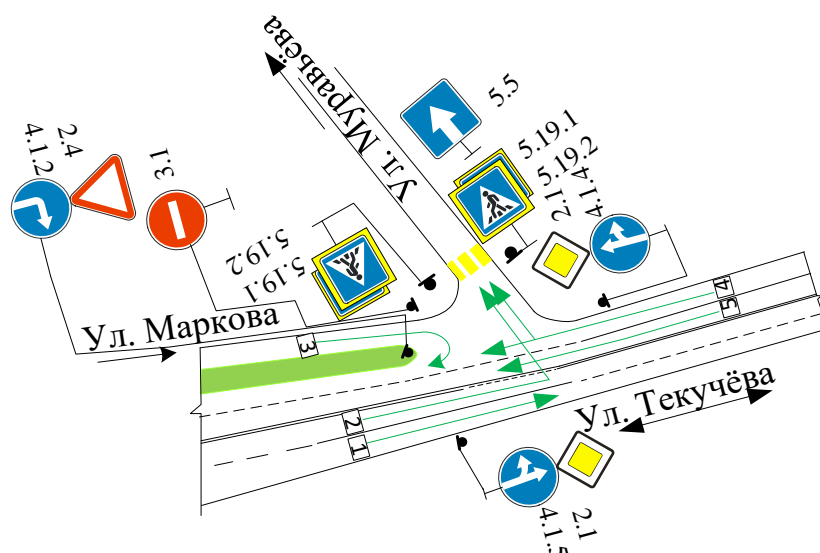
Рис. 4. Схема перекрестка «ул. Текучёва – ул. Муравьёва» с разрешенными направлениями движения
