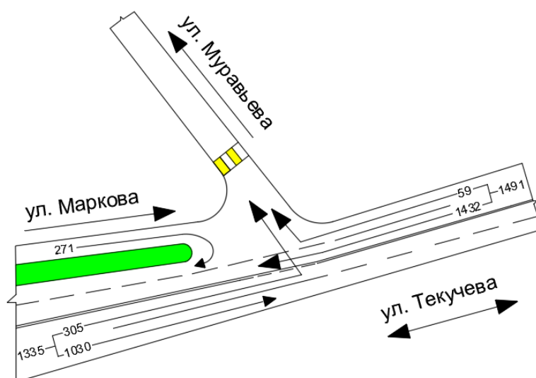
Рис. 3. Условная картограмма интенсивности движения на пересечении «ул. Текучёва – ул. Муравьёва»
