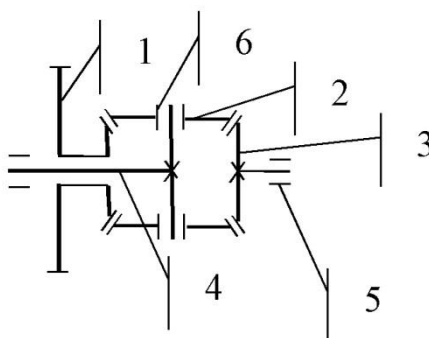
Рис. 1. Схема механического дифференциала
