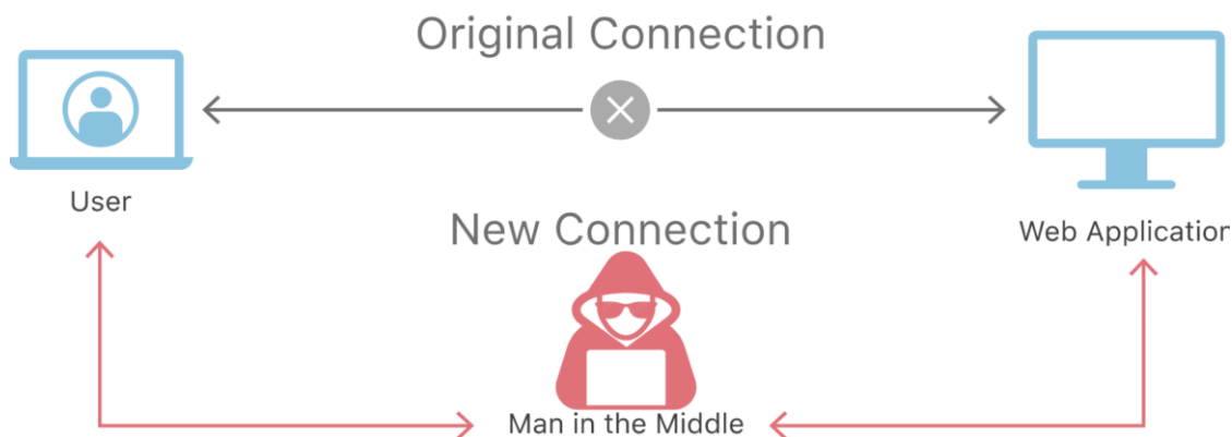
Рис. 1. Атака Man-in-the-Middle: перехват данных
