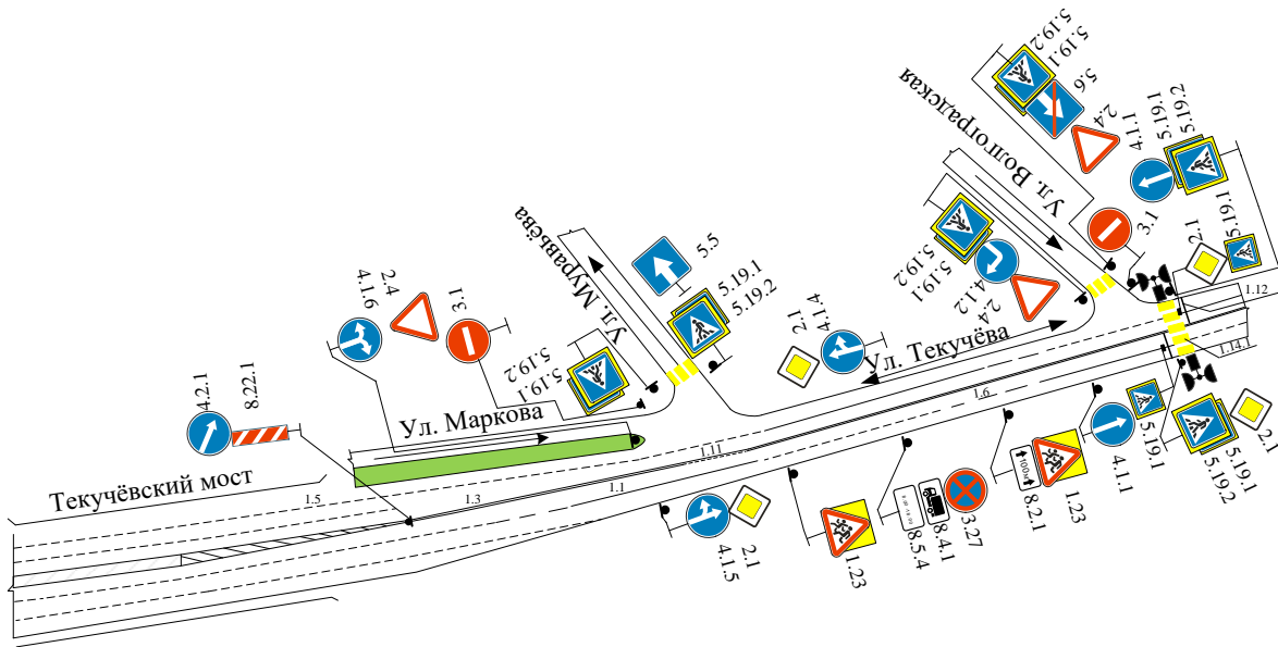
Рис. 5. Существующая схема ОДД на перегоне по ул. Текучёва от Текучёвского моста до пересечения с ул. Волгоградской
