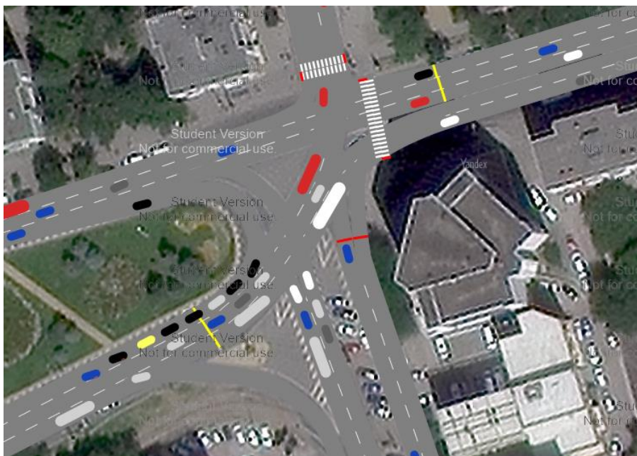
Рис. 4. Существующая модель движения транспортных средств на пересечении «ул. Красноармейская – пер. Доломановский»
