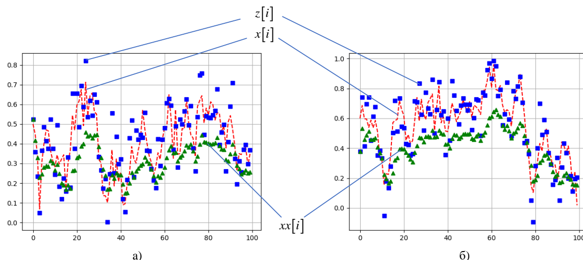
Рис. 1. Зависимость ВОСЛ между НЗС и ЛА от шага управления связи с применением фильтра Калмана: а) первое испытание, б) второе испытание, где x[l] – значение ВОЛС, рассчитываемое по моделью прогноза; z[l] – заданное значение, которое может получить из модель оценки с учетом параметров трасса связи; xx[l] – прогнозируемое значение ВОЛС на основе теории фильтрации Калмана
