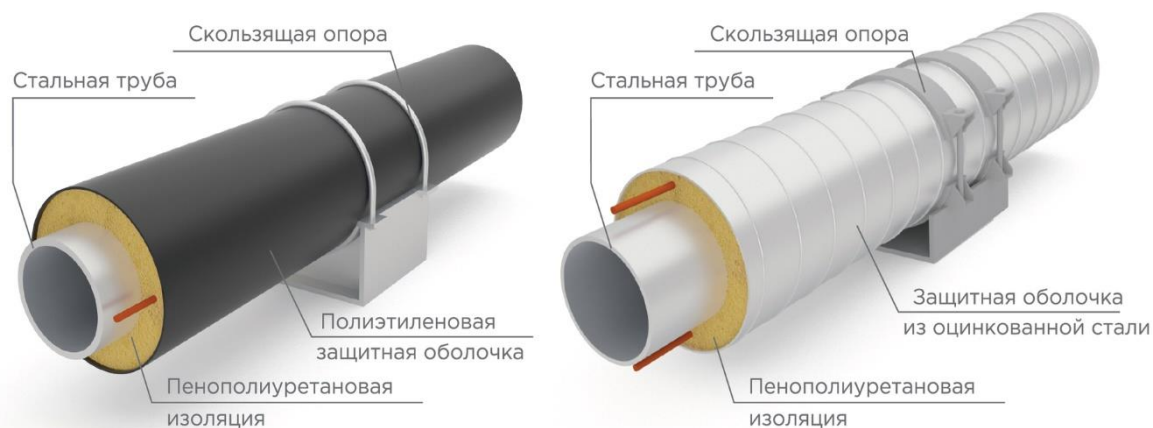
Рис. 1. Теплоизоляция трубопроводов
