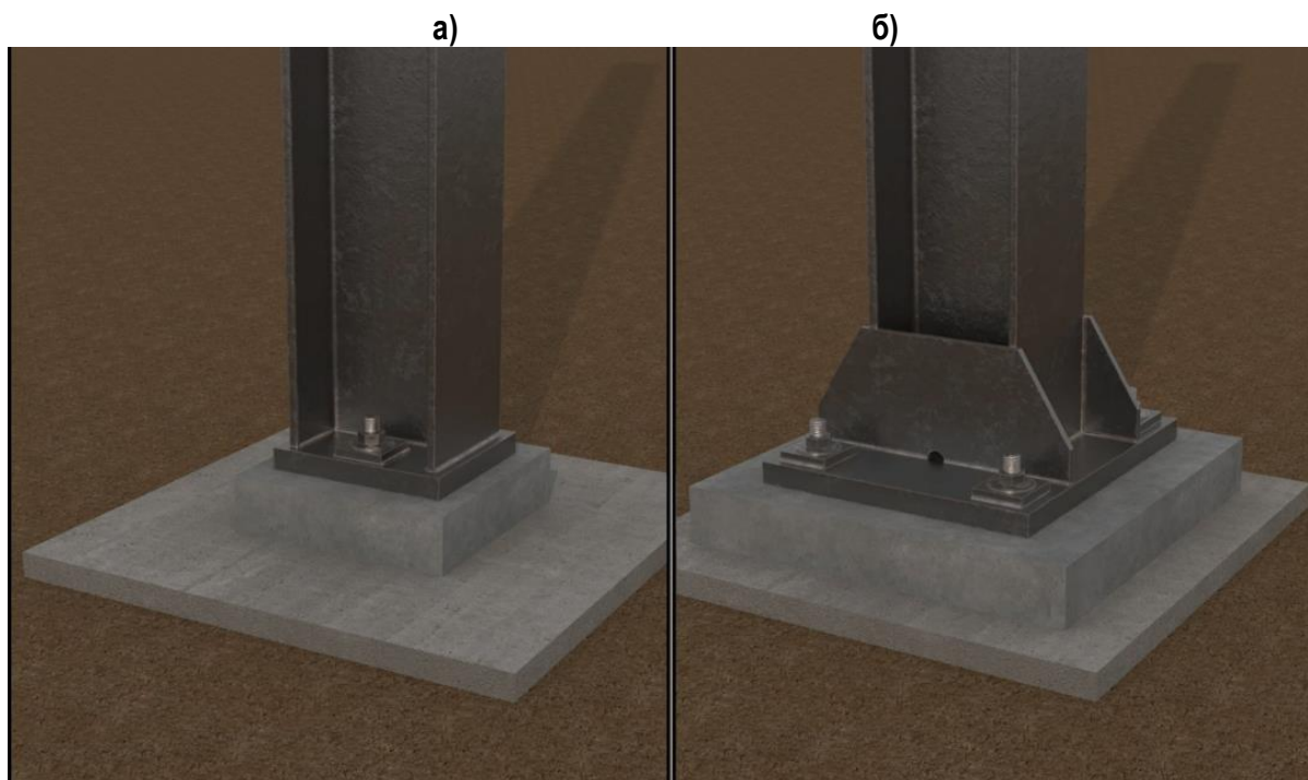
Рис. 1. Виды сопряжения колонн с фундаментами: а)- шарнирная база; б)- жесткая база
