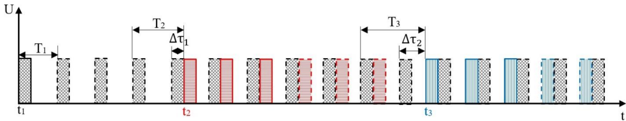
Рис. 2. Диаграмма импульсных радиосигналов на временной шкале
