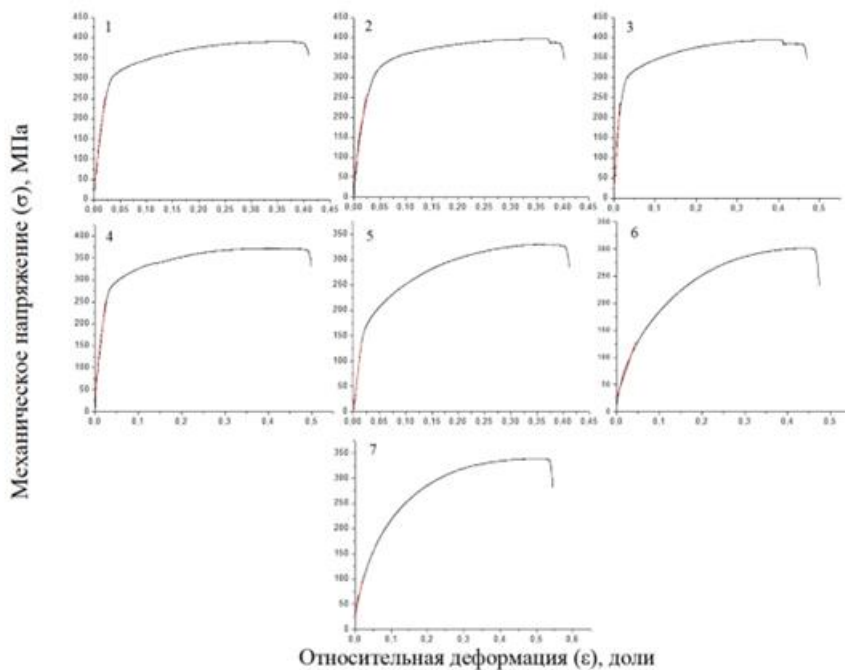
Рис. 5. Построение касательной к кривой деформации для расчета модуля Юнга при различной температуре отжига: 1 – до отжига; 2 – 100 °С; 3 – 200 °С; 4 – 300 °С; 5 – 400 °С; 6 – 500 °С; 7 – 600 °С
