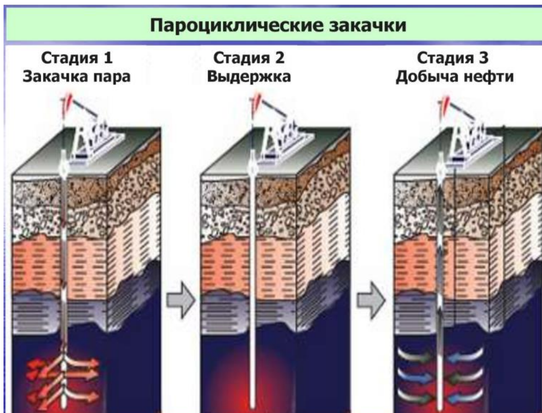
Рис. 1. Стадии пароциклической закачки
