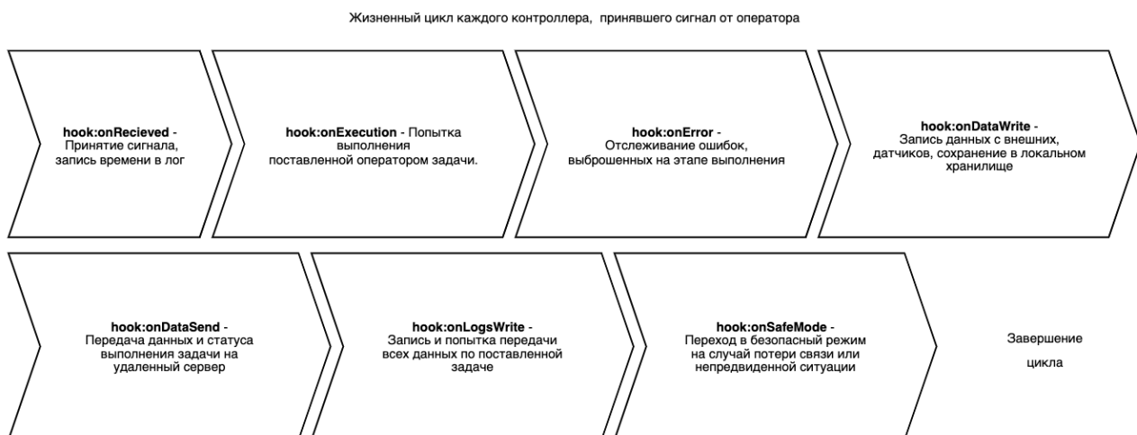
Рис. 1. Схема цикла вызова хуков на стороне контроллера
