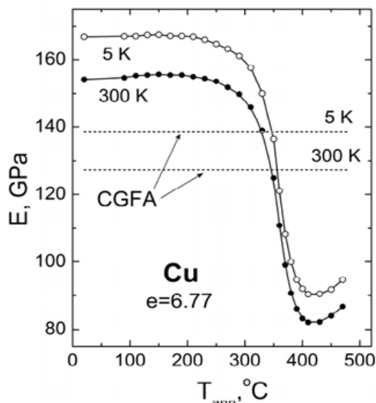
Рис. 6. Влияние температуры отжига на величину динамического модуля Юнга E при 5 К и 300 К [3]
