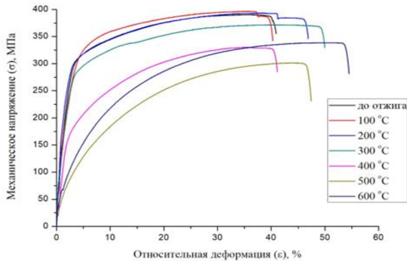
Рис. 4. Графики зависимости механического напряжения меди от относительной деформации
