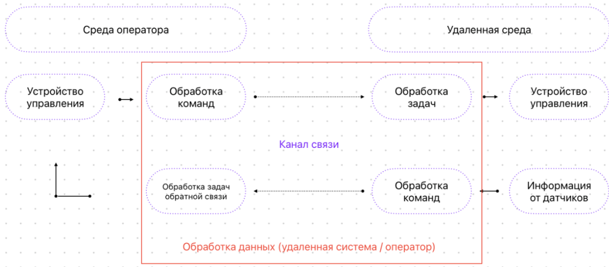
Рис. 2. Общая схема архитектуры фреймворка
