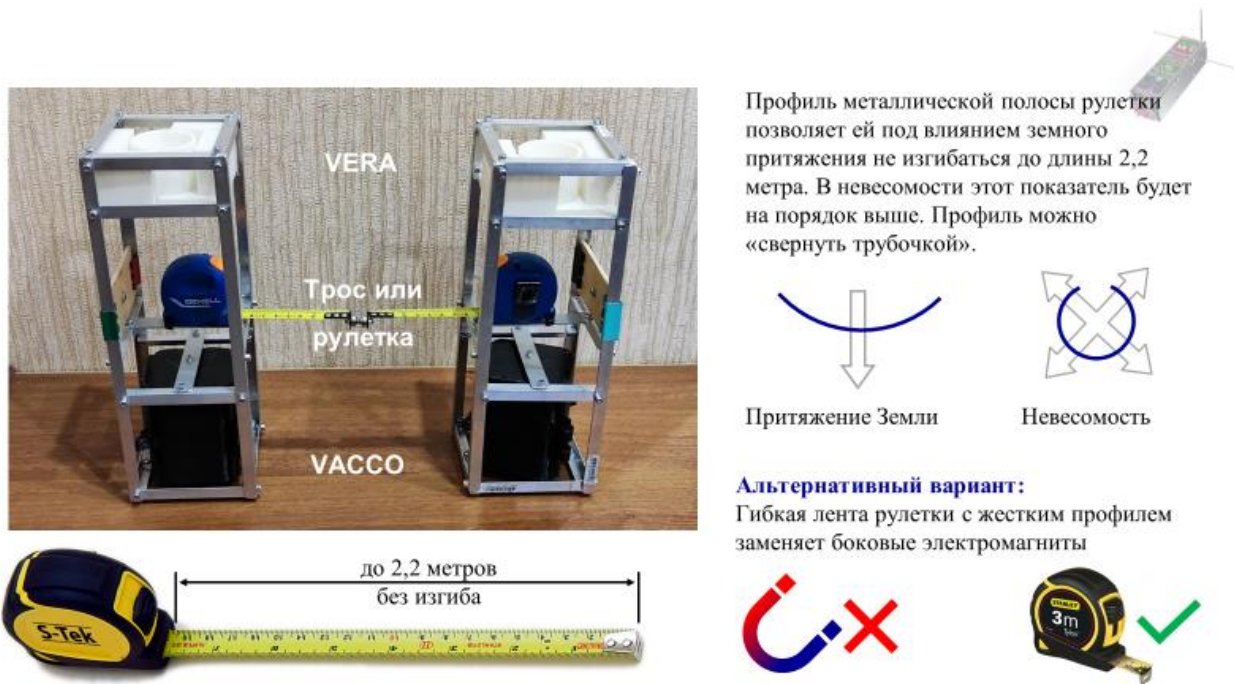
Рис. 3. Макеты кубсатов
