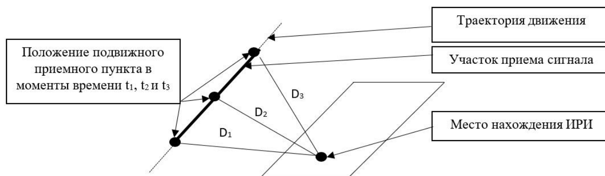
Рис. 1. Графическое отображение способа ОМП ИРИ с помощью одного подвижного приемного пункт
