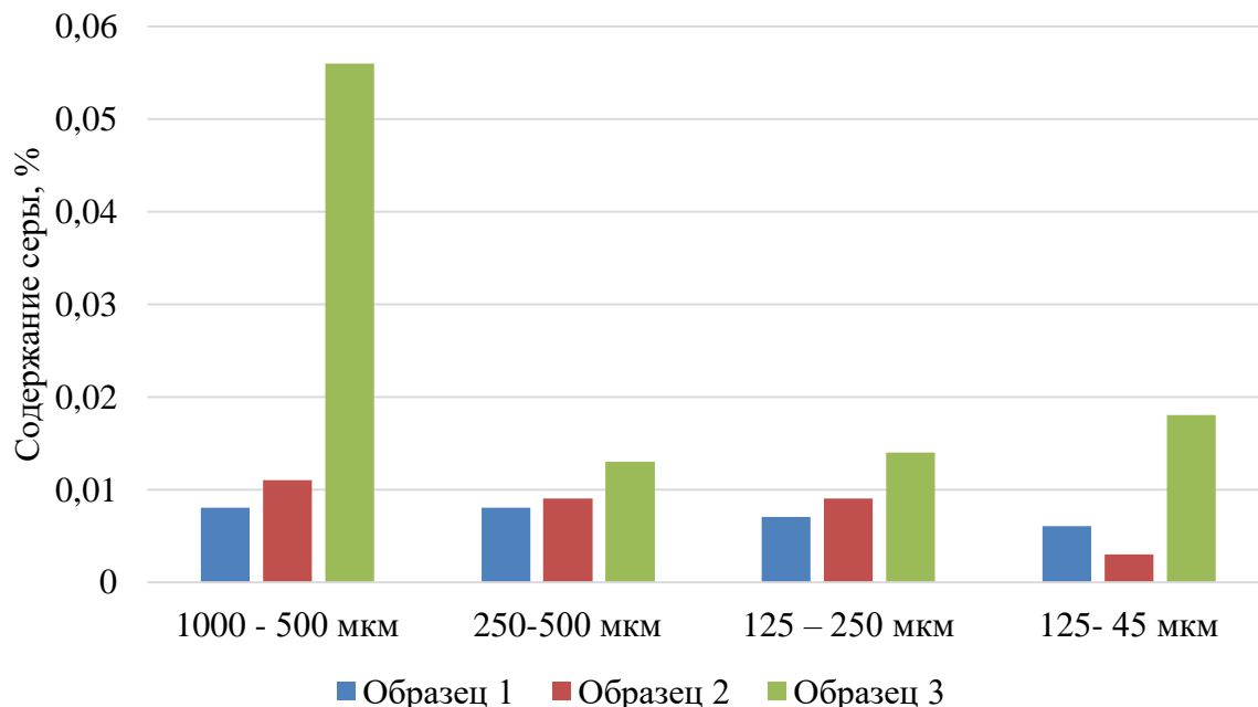
Рис. 1. Результаты исследования содержания сернистых соединений в исходных почвах
