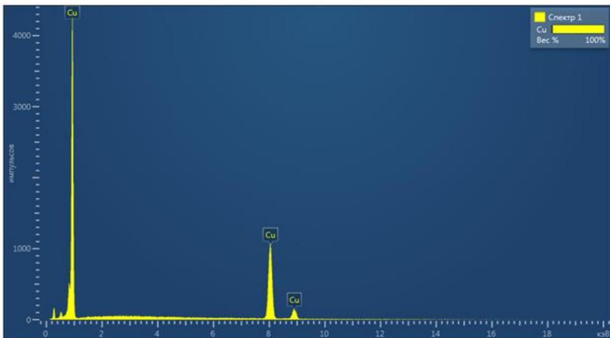
Рис. 1. Спектр характеристического рентгеновского излучения медной проволоки
