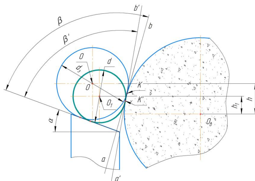
Рис. 2. Угловое смещение касательной ab в результате съема припуска
