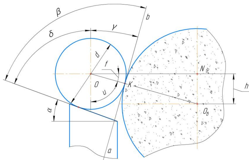
Рис. 1. Схема взаимодействия заготовки с ведущим кругом
