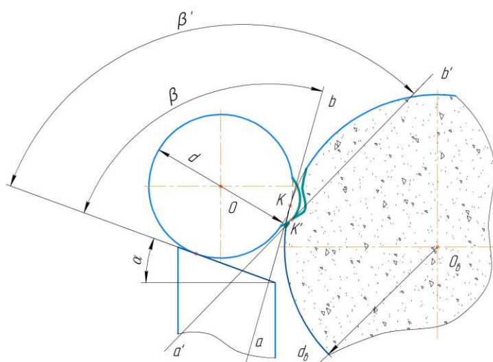
Рис. 3. Угловое смещение касательной ab при набегании неровностей обрабатываемой поверхности
