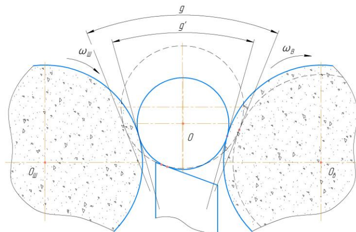
Рис. 4. Изменение угла клинового пространства между абразивными кругами
