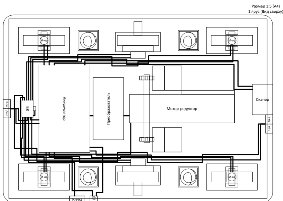
Рис. 1. Структурная схема логистического робота
