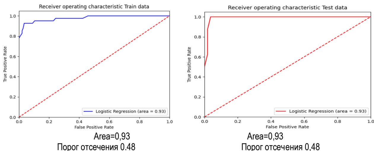
Рис. 2. Общий отчет о классификации: Обучающая – чувствительность -95%, специфичность – 95%. Тестовая -чувствительность -97%, специфичность -97%.
