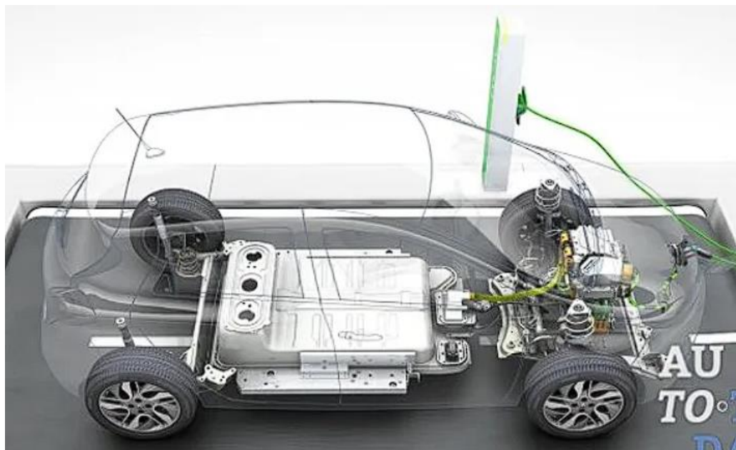
Рис. 1. Электрокар
