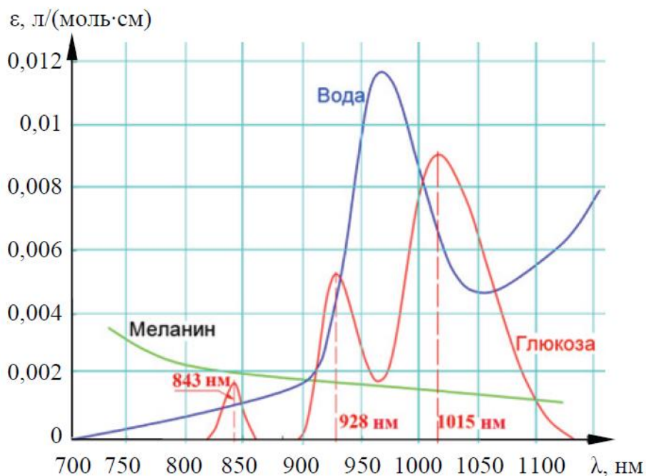
Рис. 1. Спектры поглощения воды и глюкозы в ИК-диапазоне
