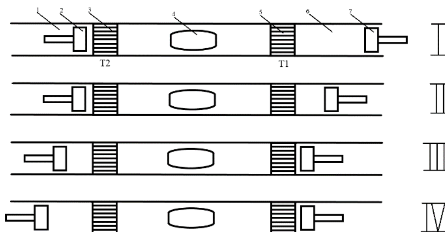
Рис. 2. Схема работы холодильной машины Стирлинга 1 – цилиндр; 2– детандерный поршень; 3 – теплообменник нагрузки (ТН); 4 – регенератор; 5 – холодильник; 6 – полость сжатия газа; 7 – компрессорный поршень
