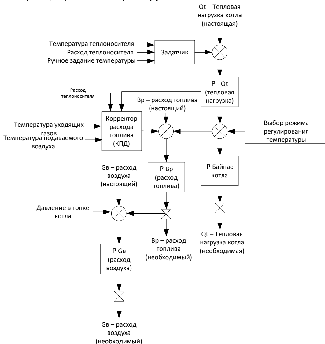
Рис. 1. Алгоритм управления и регулирования параметров котлоагрегата
