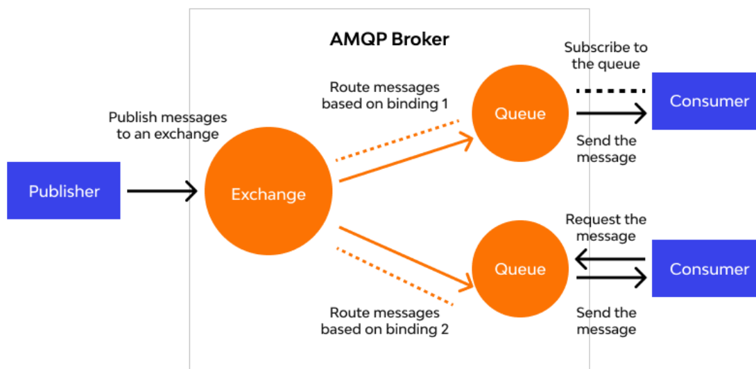
Рис. 2. Процесс обмена сообщениями в протоколе AMQP 0.9.1
