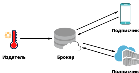
Рис. 1. Процесс обмена сообщениями в протоколе MQTT
