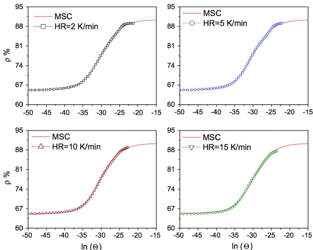
Рис. 1. Эталонные кривые спекания ThO 2 с 4% UO 2 в сравнении с экспериментальными результатами для четырех различных скоростей нагрева [8]
