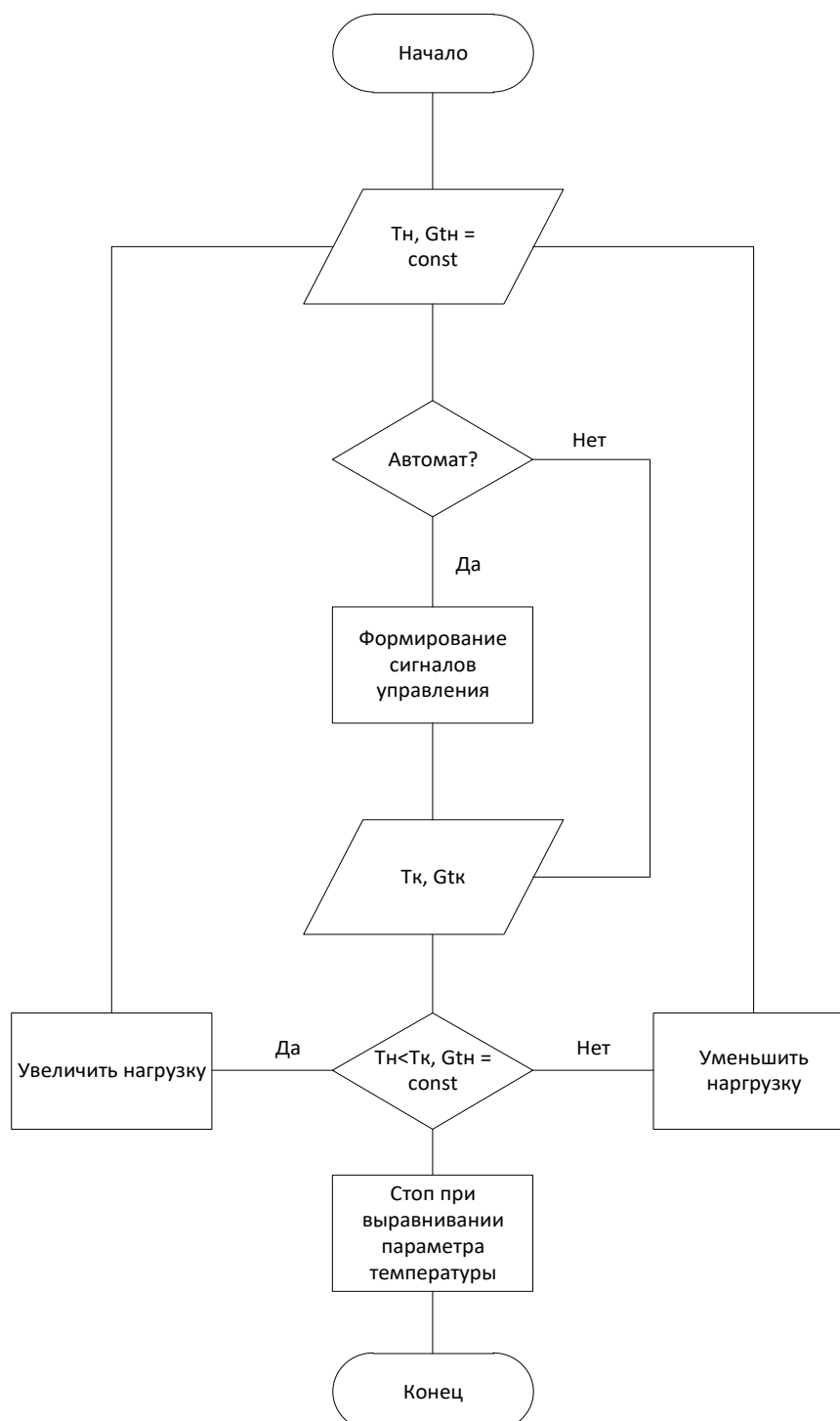
Рис. 2. Упрощенная блок схема регулятора тепловой нагрузки
