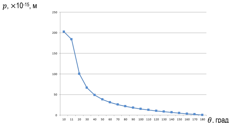
Рис. 2. Зависимость угла рассеяния \theta от прицельного параметра p
