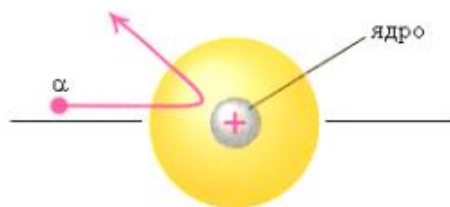
Рис. 1. Рассеяние альфа-частицы в атоме Резерфорда
