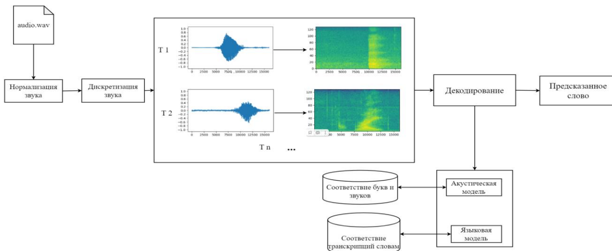
Рис. 1. Схема работы алгоритма распознавания речи Vosk
