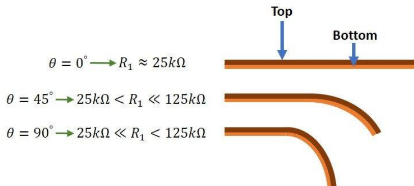
Рис. 3. Пример работы датчика Flex
