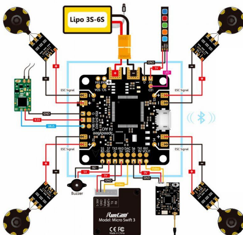
Рис. 1. Пример подключения деталей дрона к ПК
