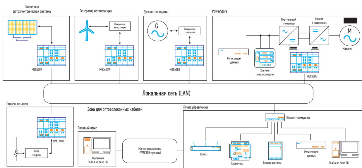
Рис. 2. Структурная схема «MicroGrid Plus»
