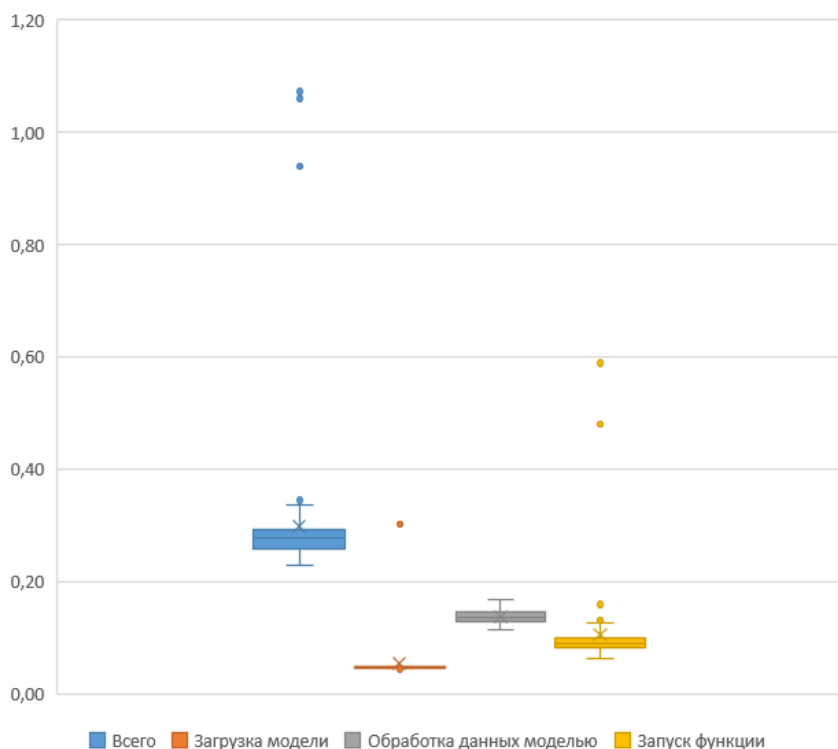
Рис. 4. Распределение времени обработки запроса функцией при загрузке модели snn3.tflite в одном архиве с функцией
