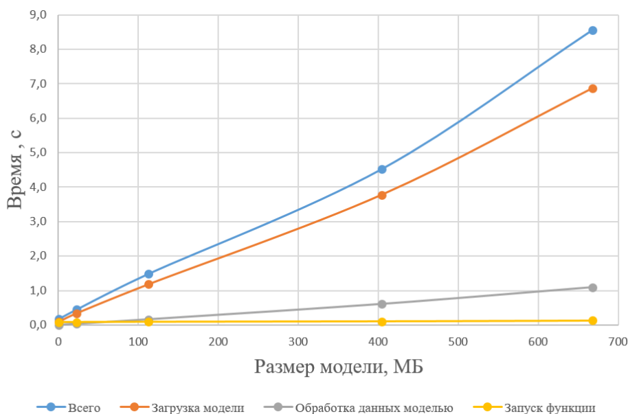
Рис. 1. График времени выполнения функции в зависимости от размера модели в облаке Yandex Cloud
