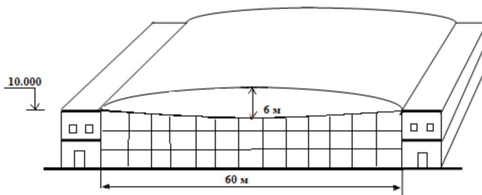
Рис. 1. Мембранно-пневматическое здание пролетом 60 метров
