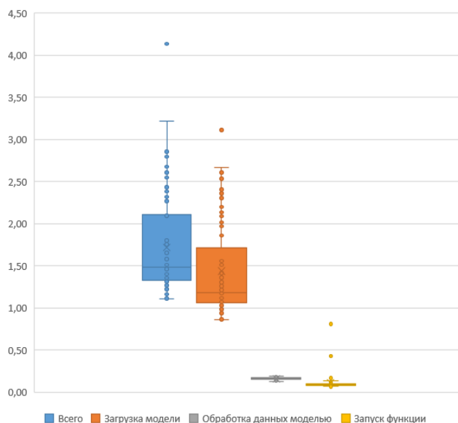
Рис. 3. Распределение времени обработки запроса функцией при загрузке модели snn3.tflite из объектного хранилища
