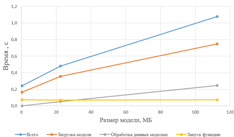
Рис. 2. График времени выполнения функции в зависимости от размера модели в облаке Selectel
