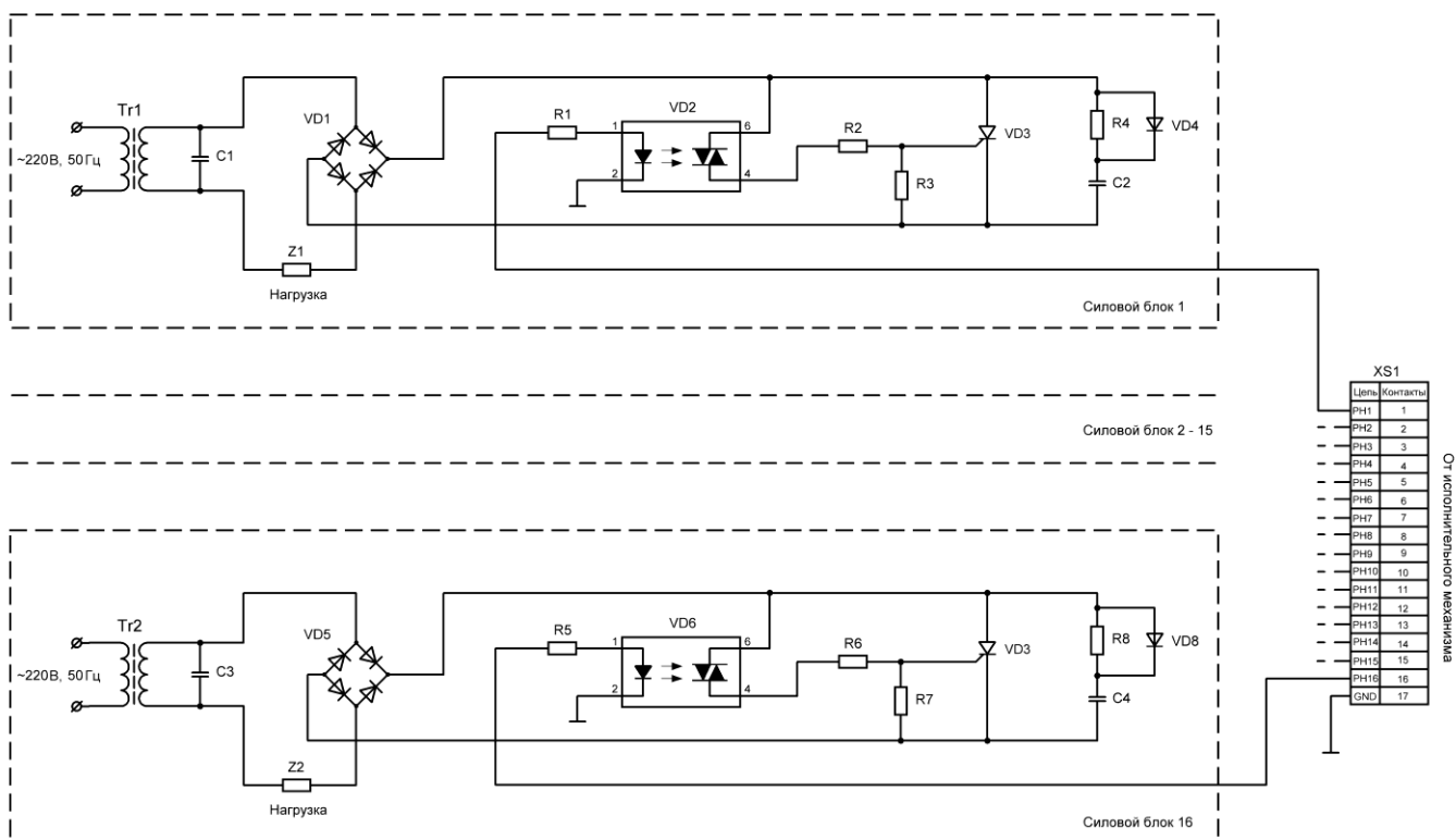
Рис. 1. Принципиальная электрическая схема разработанной силовой части регулятора напряжения
