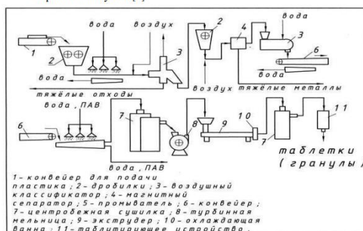
Рис. 2. Процесс создания материала для дорожного покрытия
