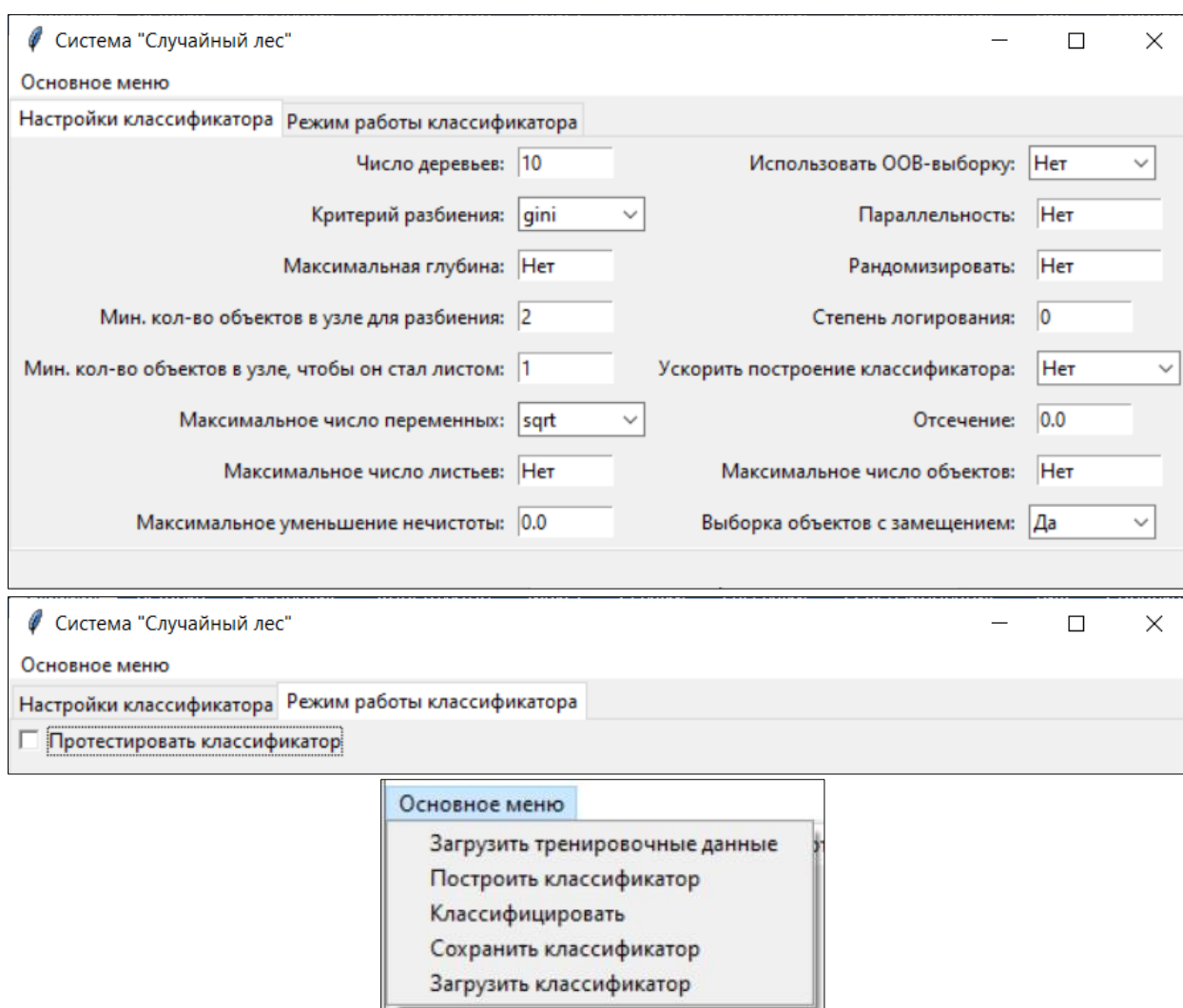
Рис. 1. Система «Случайный лес». Интерфейс пользователя
