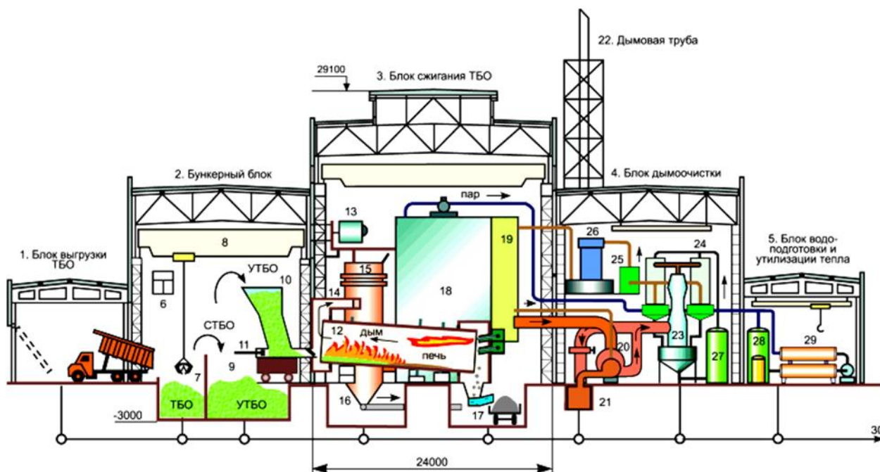
Рис. 2. Котельная установка
