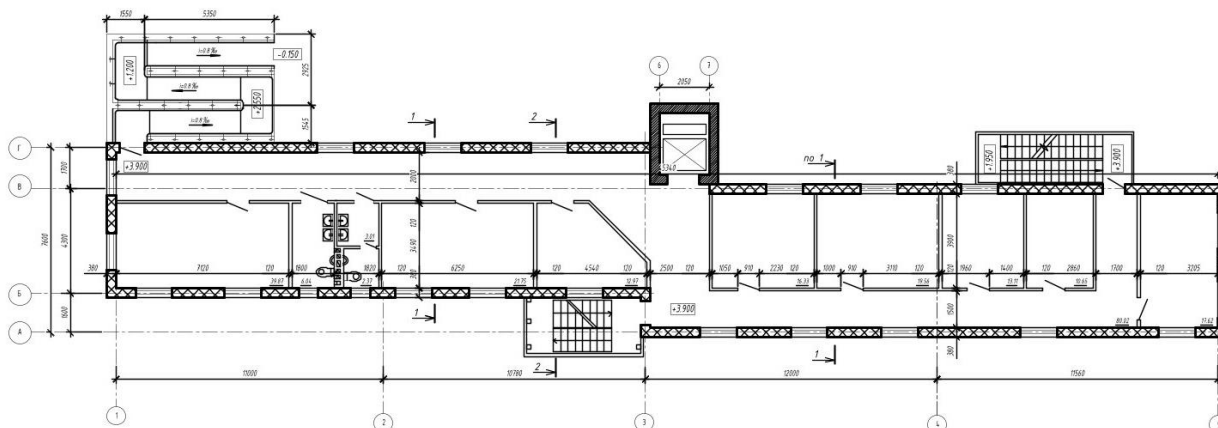
Рис. 4. План 2-го этажа после реконструкции
