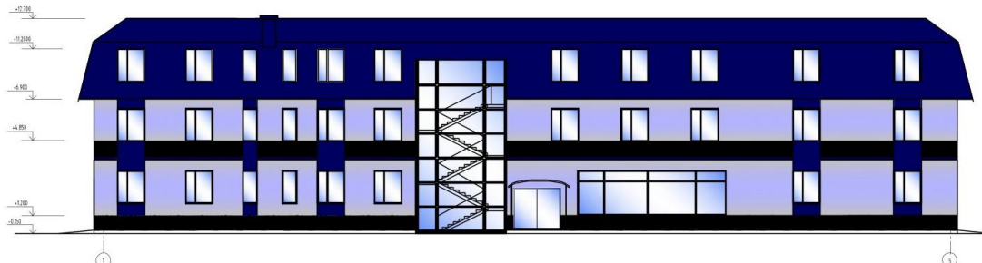
Рис. 2. Фасад после реконструкции
