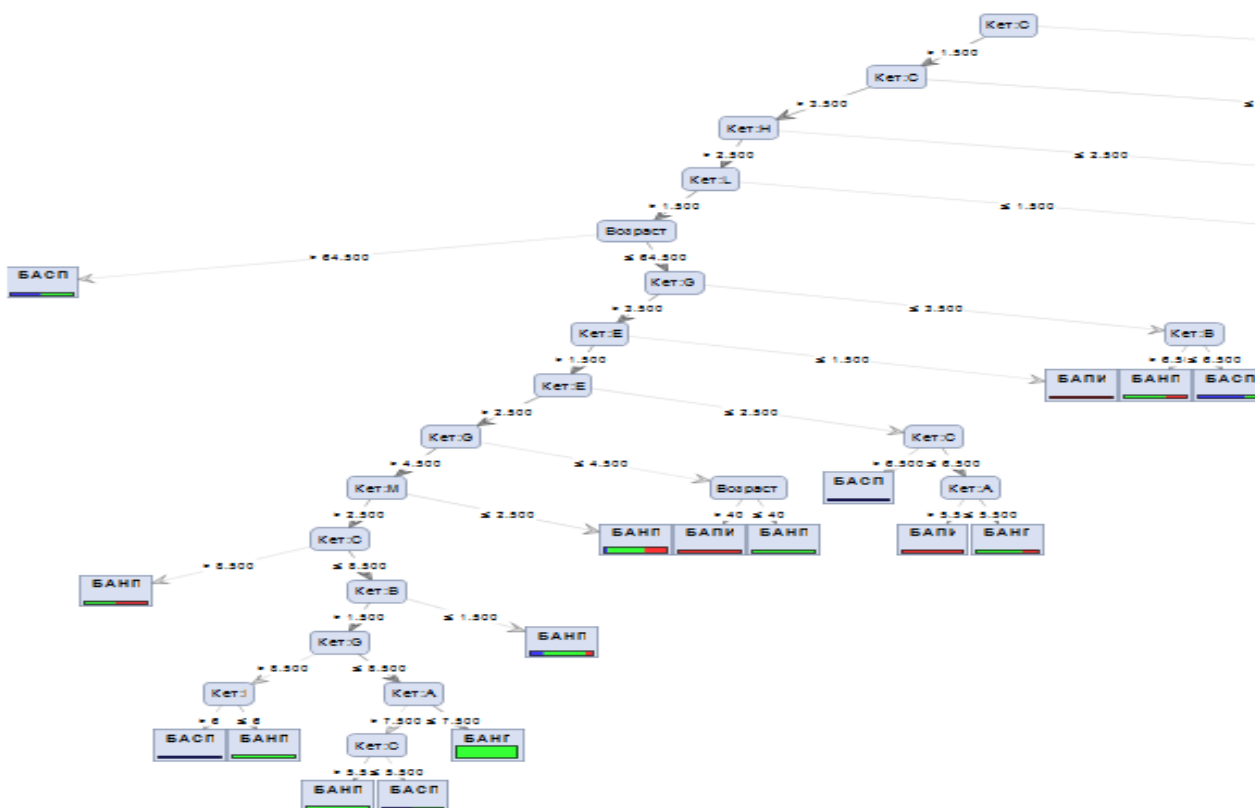
Рис. 1. Дерево решений
