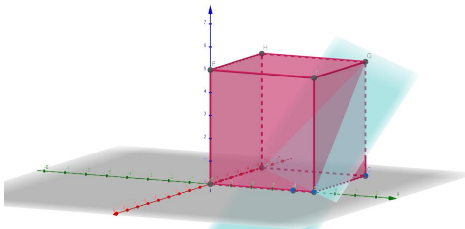
Рис. 1. Наглядный пример построения сечения в ресурсе GeoGebra
