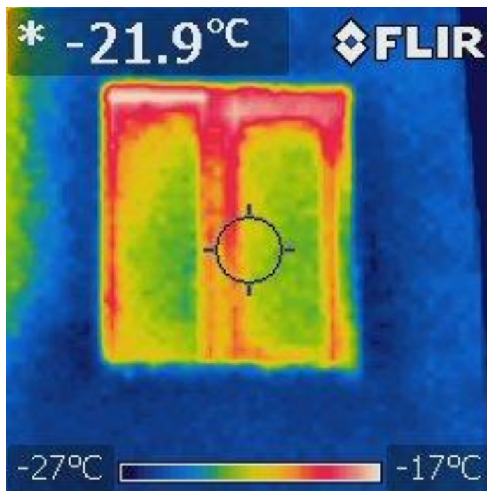
Рис. 2. Тепловизионная съемка стены с низкими тепловыми потерями
