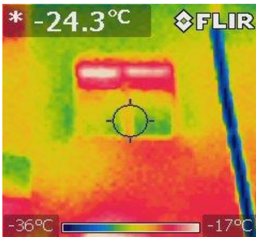
Рис. 1. Тепловизионная съемка стены с высокими тепловыми потерями
