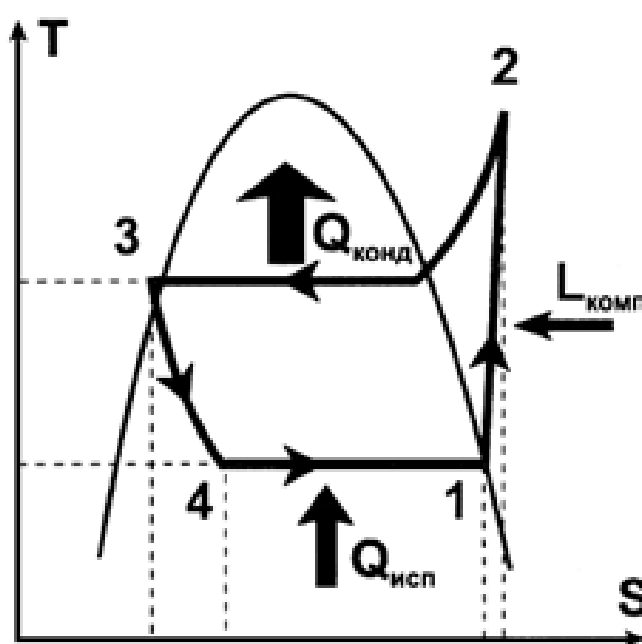
Рис. 1 T-s диаграмма
