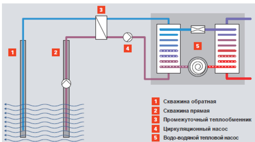
Рис. 3. Принципиальная схема теплового насоса типа «вода – вода»
