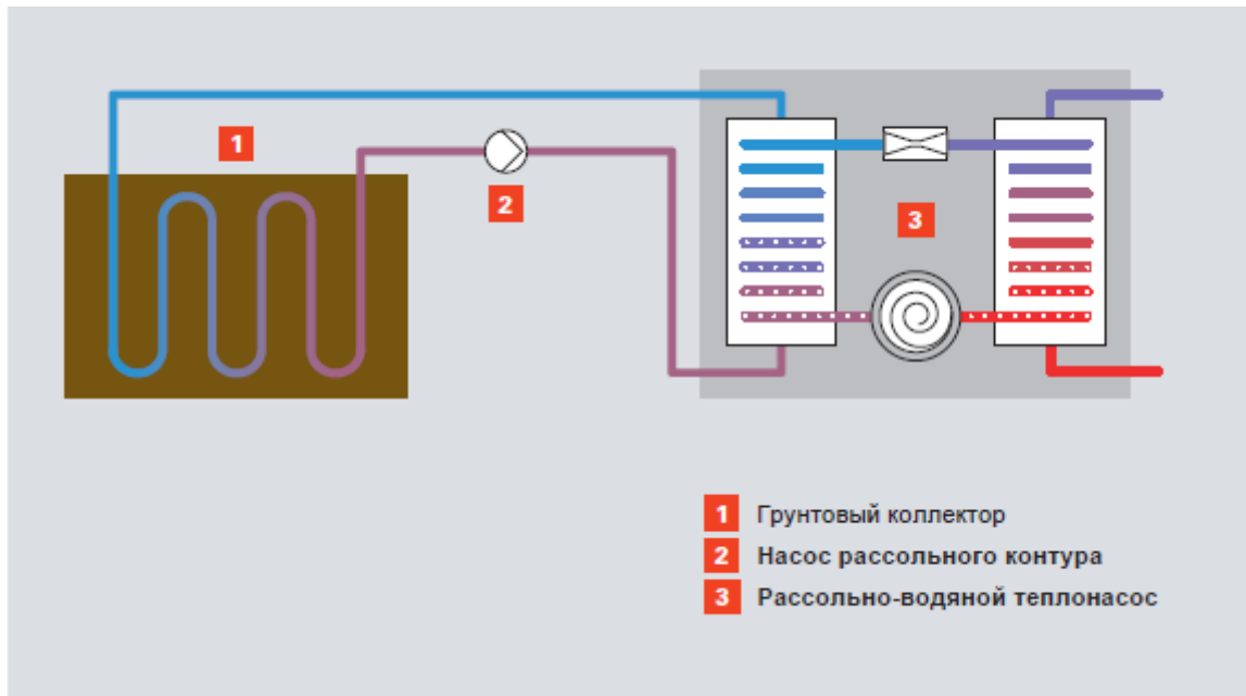
Рис. 2. Принципиальная схема теплового насоса типа «грунт—вода» с источником тепла – грунтовый коллектор
